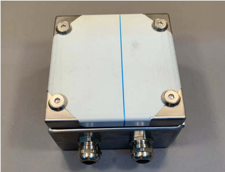
图 1 测试样品 (1#)
